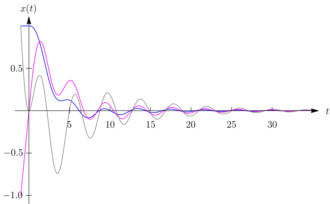
Рисунок 4: Решения системы (6.12) при \omega_1 = 1 , \omega_2 = \sqrt{3}
