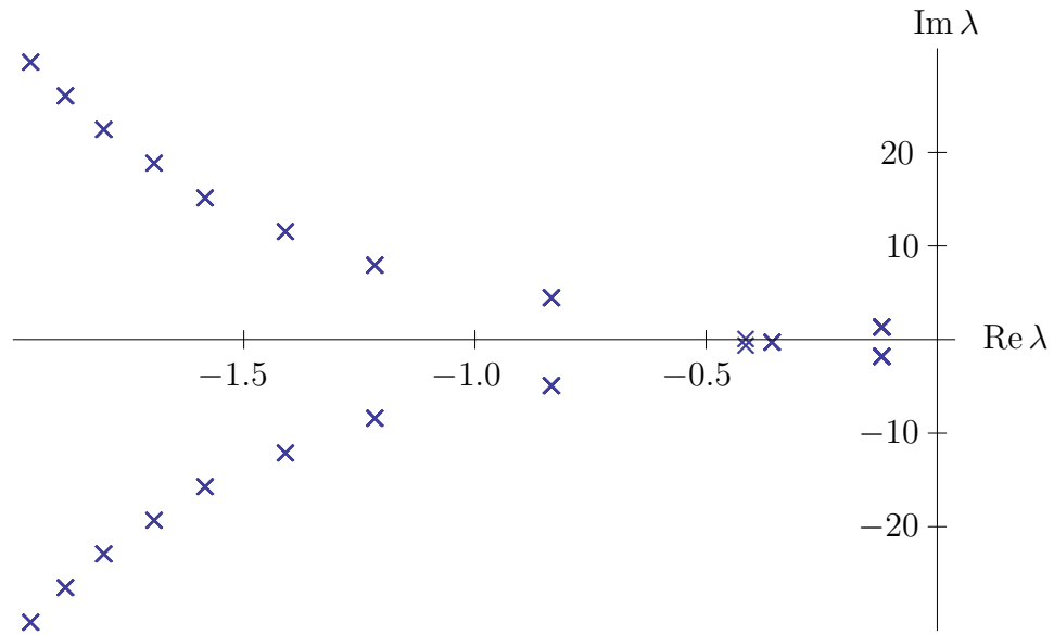
Рисунок 3: Спектр системы (6.12) при \omega_1 = 1 , \omega_2 = \sqrt{3}
