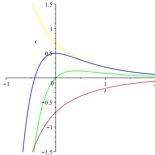
Рисунок 5: Решения системы (19.49)
