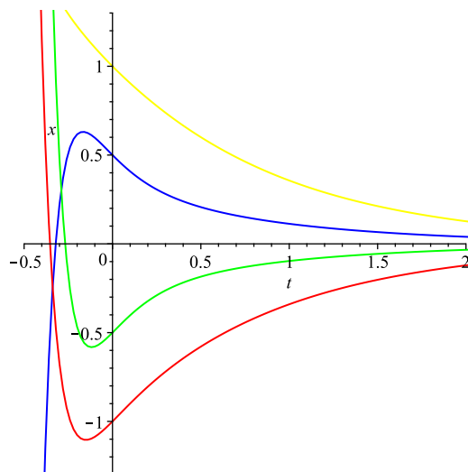
Рисунок 6: Решения системы (20.22)
