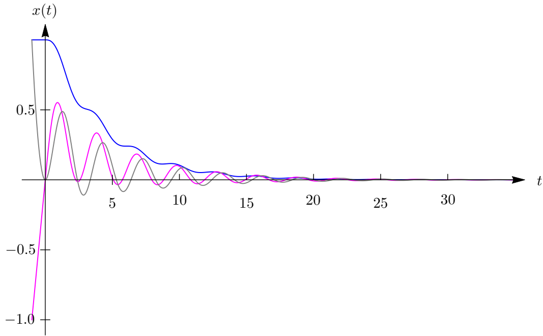
Рисунок 2: Решения замкнутой системы (6.6) при различных начальных условиях
