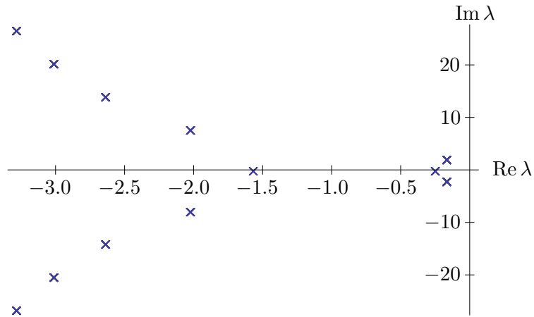
Рисунок 1: Спектр замкнутой системы (6.6) при h = 1
